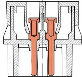
Krimp Bağlantı
