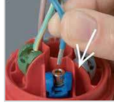
1) Kabloyu takın
