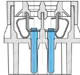
Yaylı Bağlantı
