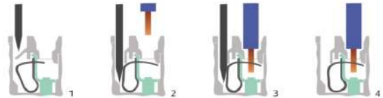
Yaylı Bağlantı
